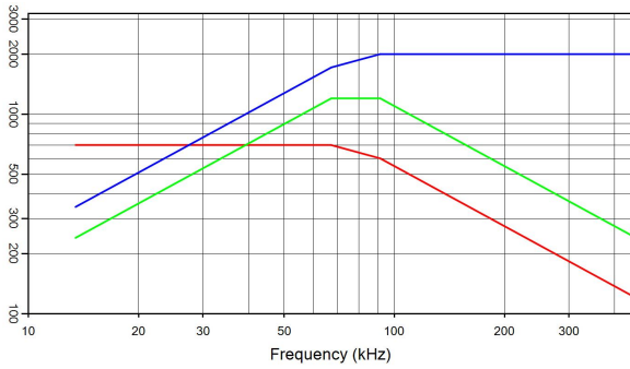
C-CAP 04 5.8 µF 700 V rms 2000 A rms 1200 kVA r I(A) — Q(kVA r ) — V rms —
