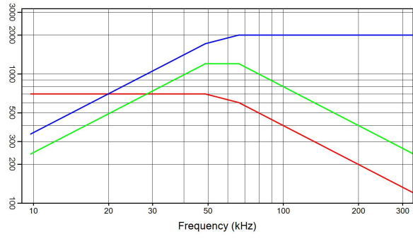
C-CAP 04 8 µF 700 V rms 2000 A rms 1200 kVA r I(A) — Q(kVA r ) — V rms —
